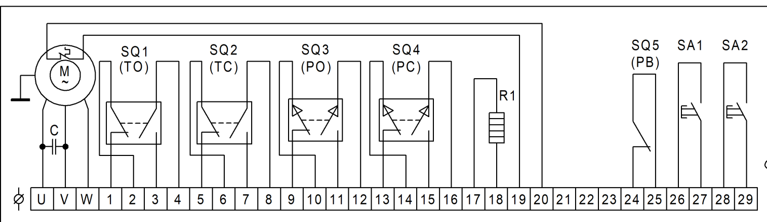
Схема электрическая соединений CE213-5C AC 230В 50Гц
